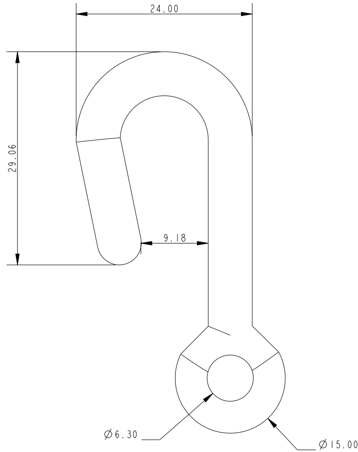
SCALE 2:1
