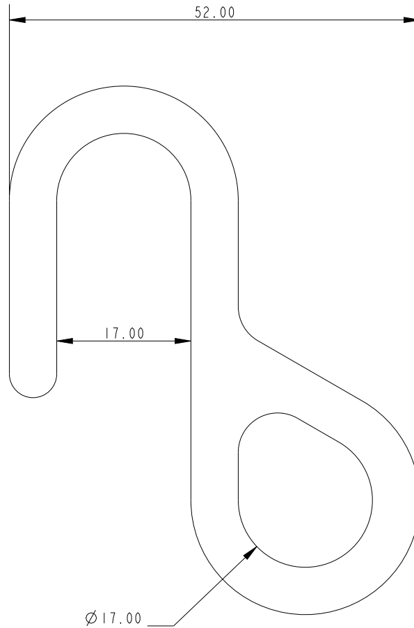
SCALE 3:2
